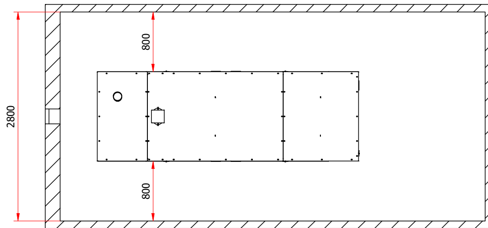
A-A ( 1 : 50 )
