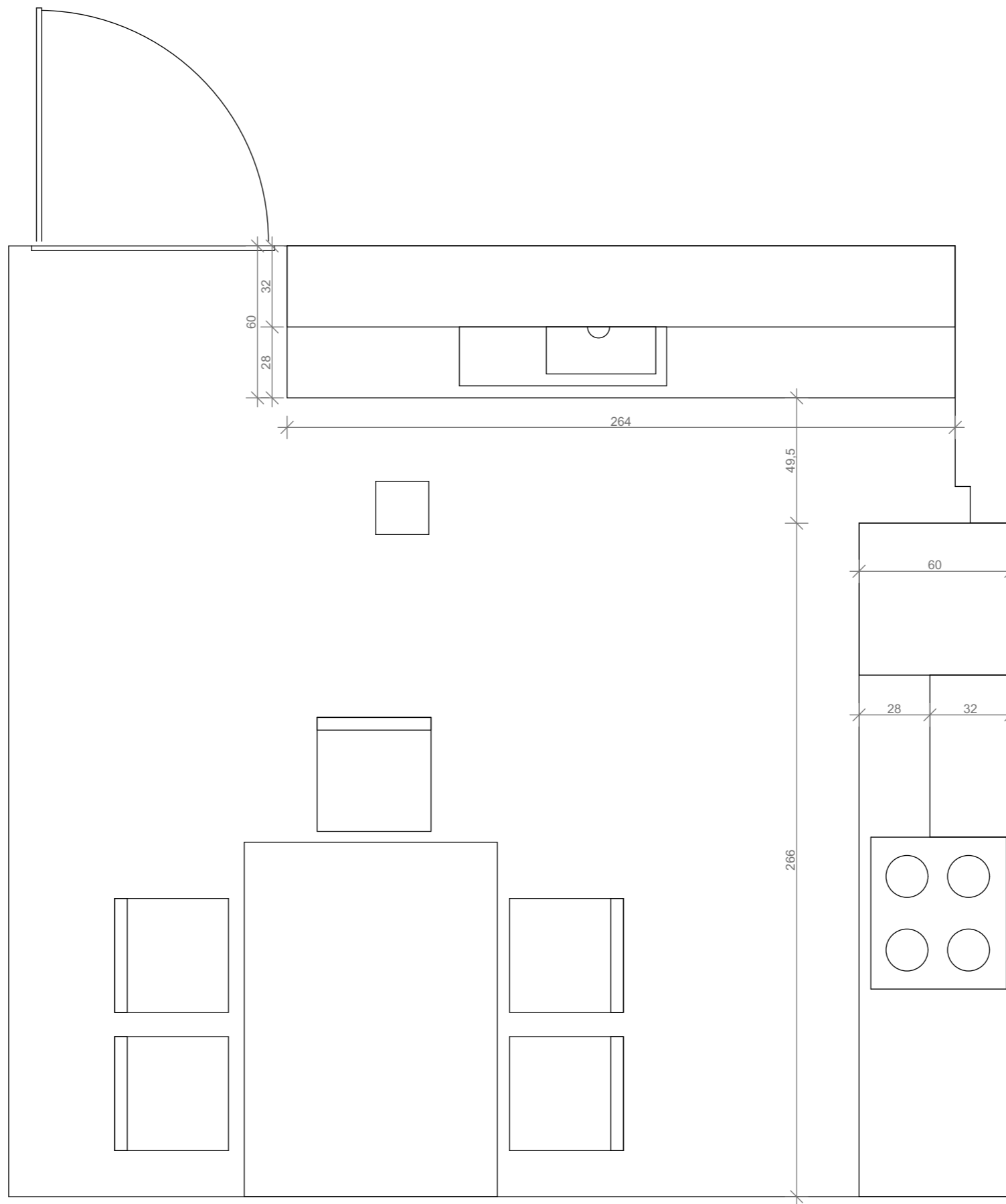
Kuchnia rzut
