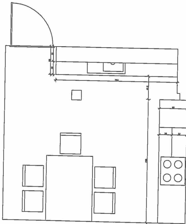
Kuchnia rzut
